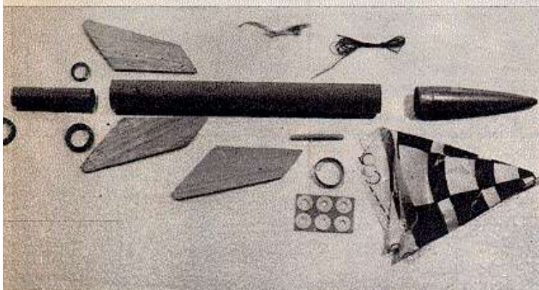
1 Piezas que componen el "Astro". Los materiales son: cartón, madera balsa, plástico, hilo y goma.
