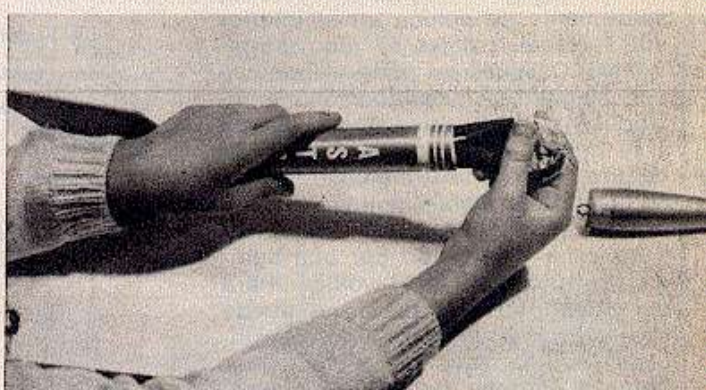
5 A continuación, perfectamente plegado se introduce en el fuselaje el pequeño paracaídas.
