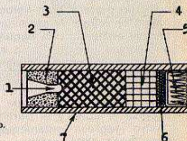
6 La ilustración muestra claramente en qué consiste un impulsor modelo. El A8-6 es similar.
