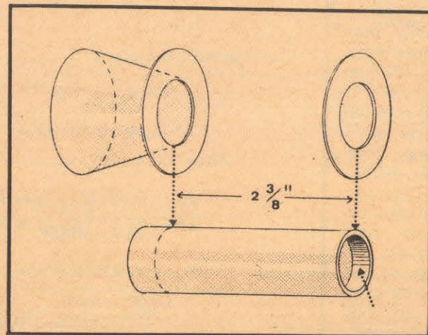
Cómo se arma la celda que contendrá el propulsor y a la cinta de freno.
