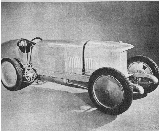
Este es el famoso Blitzen Benz con el cual B. Ottfield batió el record mundial de velocidad en 1910 alcanzando una máxima de 211,4 Km/h. Su motor de cuatro cilindros en línea y 21.500 cc desarrollaba 200 HP.
