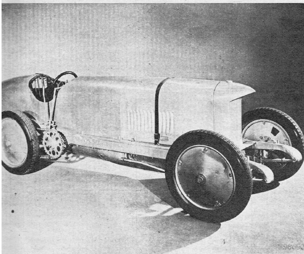
Este es el famoso Blitzen Benz con el cual B. Oldfield batió el record mundial de velocidad en 1910 alcanzando una máxima de 211,4 Km/h. Su motor de cuatro cilindros en línea y 21.500 cc desarrollaba 200 HP.
