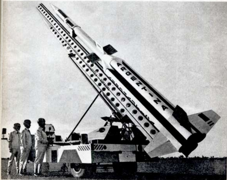
Castor: un vehículo sonda de dos etapas capaz de superar los 450 km. de altura con una carga útil de 50 kgs. Representa el máximo esfuerzo argentino en cohetoría.
