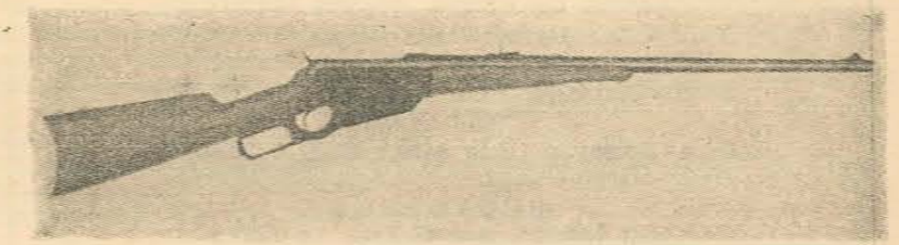
Versión desmontable de rifle Winchester 1895, para uso deportivo. La recámara fue construida más ancha en la parte superior y se le introdujeron algunas modificaciones en la parte inferior. Se le modificó la palanca, diseñándole un asa de dos piezas, para obtener un mejor cierre, se le acortó el cañón y se fabricaron modelos desmontables o comunes.
