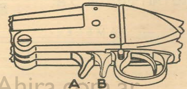
FIGURA 1. - Para obtener el cierre de la escopeta BRENTA, el gatillo suplementario de la palanca de cierre, debe encontrarse en la posición B, si se halla en la posición A o intermedia, el percutor no pegará con fuerza en el fulminante del cartucho, impidiendo el disparo.
