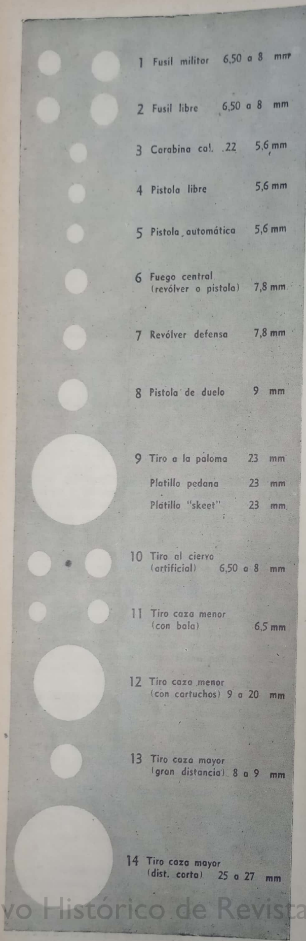
Esquemas de los distintos calibres utilizados en las distintas especialidades del deporte del tiro.
