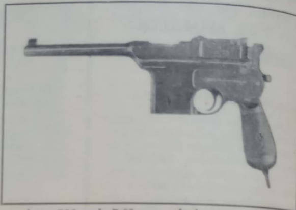
Astra 900, cal. 7,63 mm., de las primeras series, con pequeña anilla en el martillo. Posee una sola línea de inscripción: "Astra" automatic pistol cal. 7,63 mm.". Tiro semiautomático solamente.
