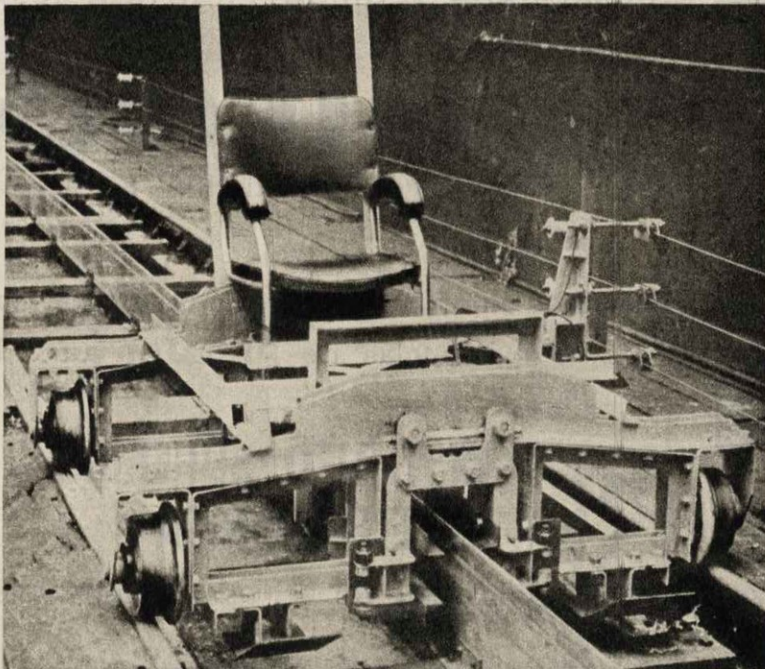
He aquí una versión experimental del motor de inducción lineal: Está montado sobre una zorra y se utiliza para sus demostraciones.
