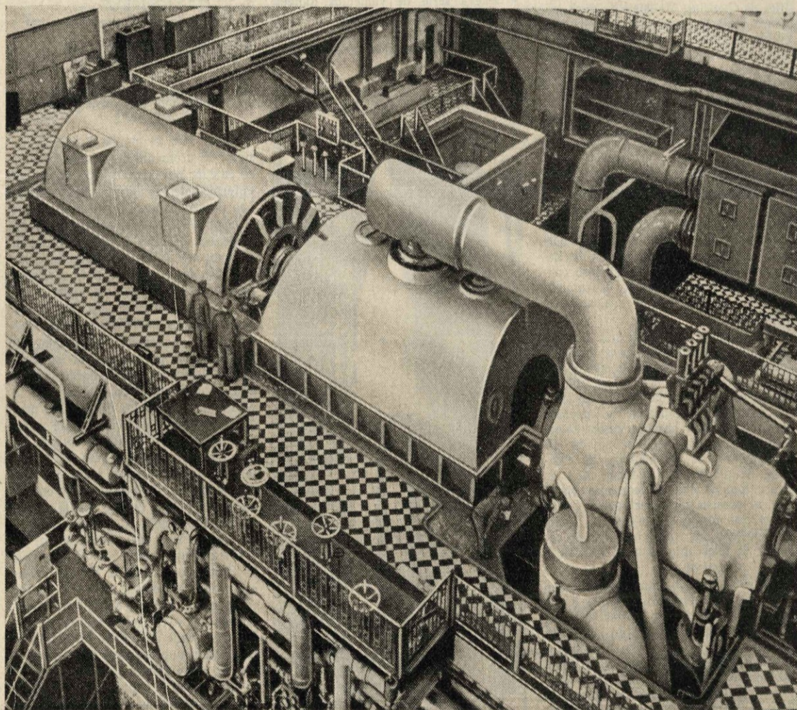
Vista del turbogenerador N° 8 de 194.000 kW de la Central Puerto Nuevo ...ES UNICO EN SUDAMERICA!
