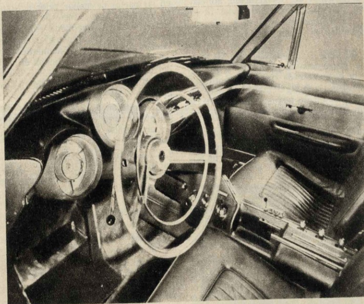
Interior del automóvil a turbina de gas, producido por Chrysler Corporation , que será presentado en Buenos Aires el próximo verano.
