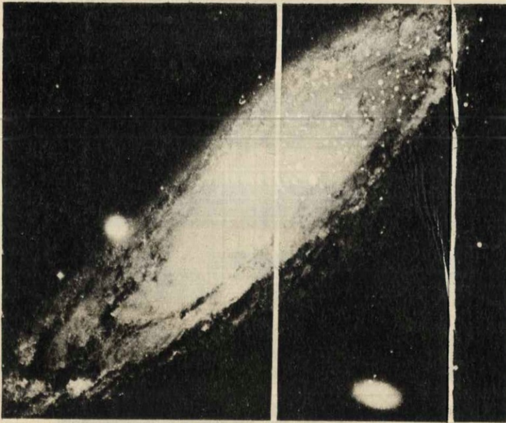
La nebulosa de Andr6meda (izq.), tal como se observa con un telescopio corriente; a la derecha, c6mo se veria con un detector de neutrinos.
