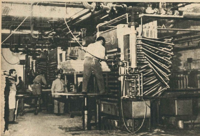
Un sector de la sección prensado, en la fábrica de Zárate, donde los pisos resilientes Sektalon empiezan a asumir su forma definitiva.
