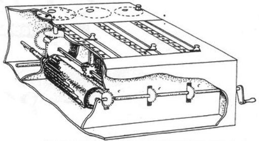
Diagrama que muestra un corte de la máquina de calcular de Leibniz
