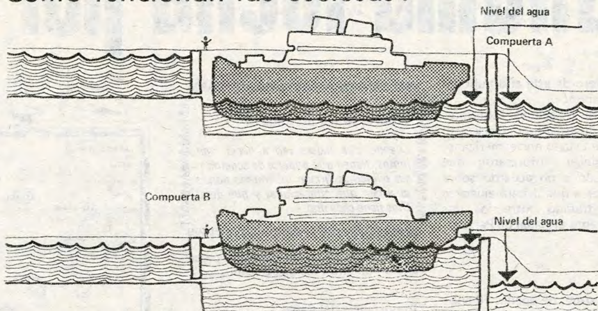
El barco entra a una esclusa. Detrás de él se cierra la compuerta A. Se llena la esclusa hasta llegar al nivel de agua de la esclusa siguiente. Se abre la compuerta B y el barco pasa.
