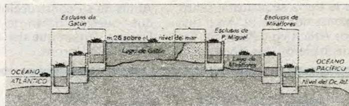
El barco entra a una esclusa. Detrás de él se cierra la compuerta A. Se llena la esclusa hasta llegar al nivel de agua de la esclusa siguiente. Se abre la compuerta B y el barco pasa.
