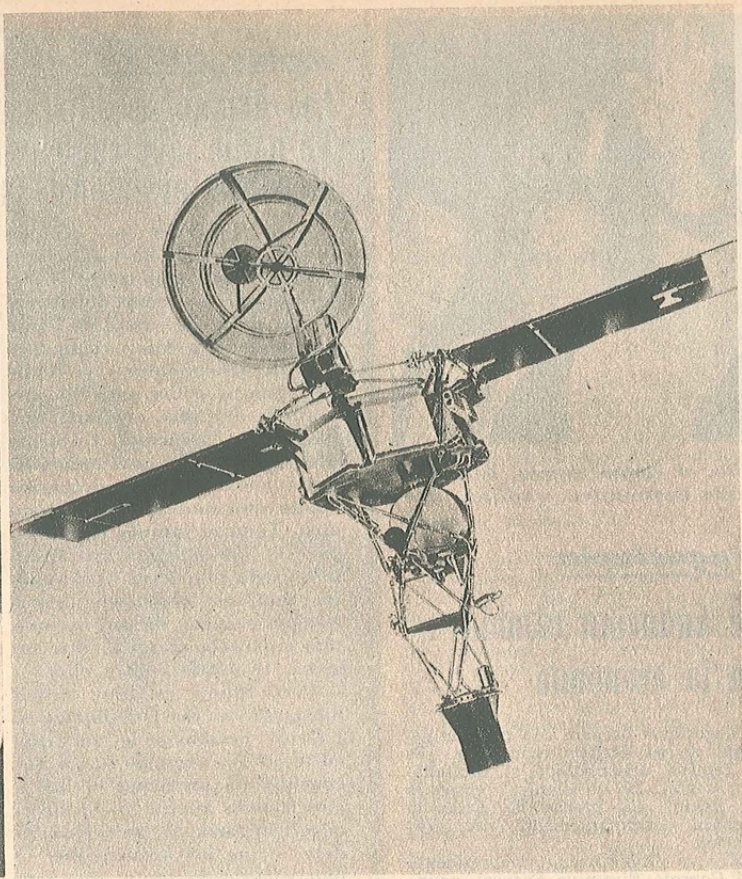
La nave espacial norteamericana, Mariner II, momentos antes de ser colocado sobre el cohete impulsor Atlas, a la izquierda; a la derecha, el Mariner con sus paneles solares desplegado y su antena de alta ganancia.
