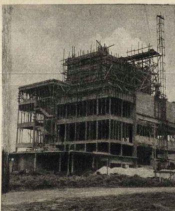
El reactor RA3, de tipo pozo, se construye en el Centro de Ezeiza.
