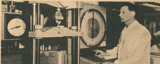
Máquina de Riehle, que desarrolla hasta 30.000 kilogramos de tensión para determinar la resistencia de las piezas del Falcon.
