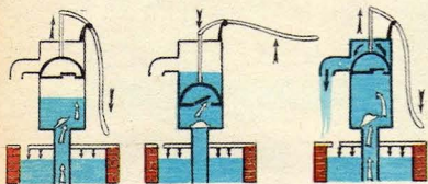
ASPIRACIÓN
