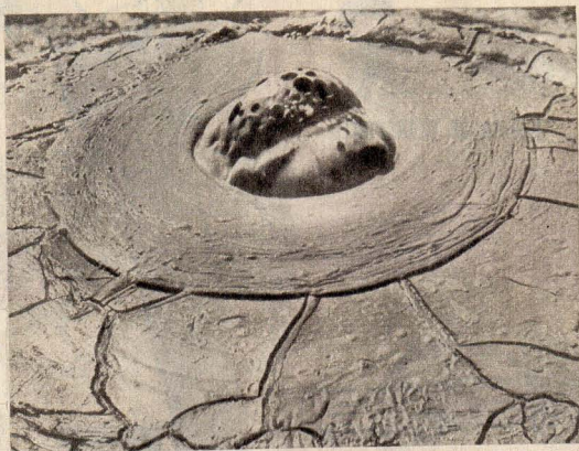
Este es el cráter del pequeño volcán Puntagorda. En el centro pueden observarse las burbujas.
