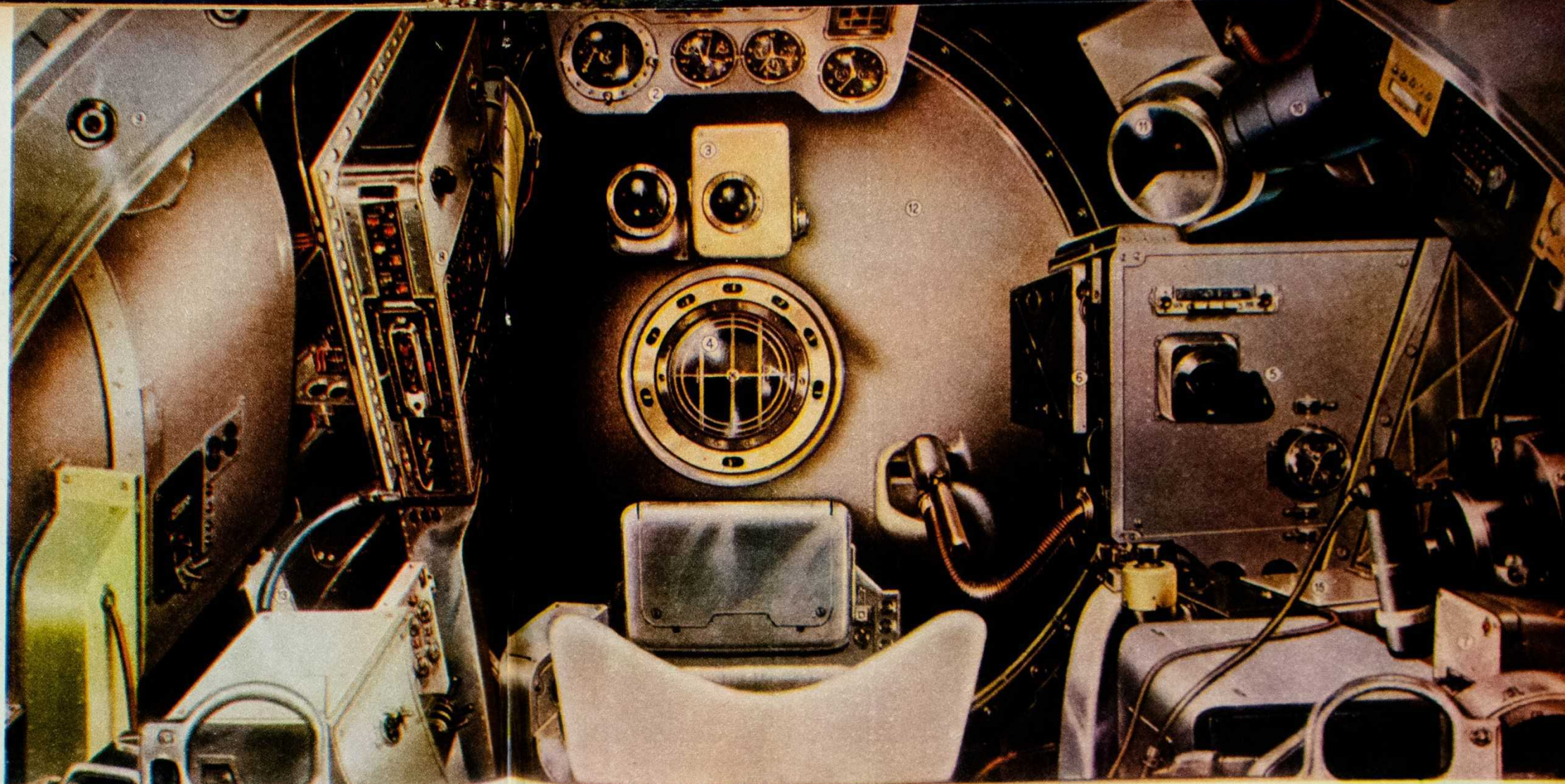
3: cámaras TV; 4: visor para observación de Tierra; 5: mandos; 6: alimentos; 9: mandos de la escotilla; 10: batería; 11: cámara.
