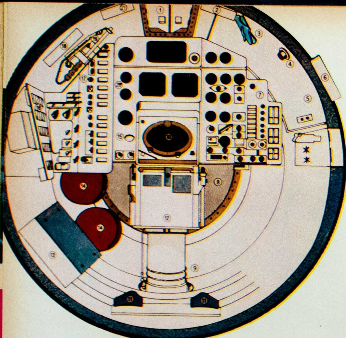
Habitáculo Mercury. 1: ventana superior; 2, 18 y 21: luces; 3: seguro de la puerta; 4 y 5: alarmas; 8: puerta de escape; 9 y 12: periscopios; 10: visor; 11: pedales; 13: alimentos; 14: aire; 7, 15, 16, 17 y 26: controles.
