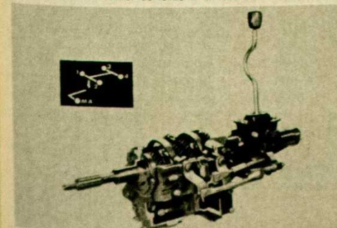
Caja ZF de 4 marchas sincronizadas
