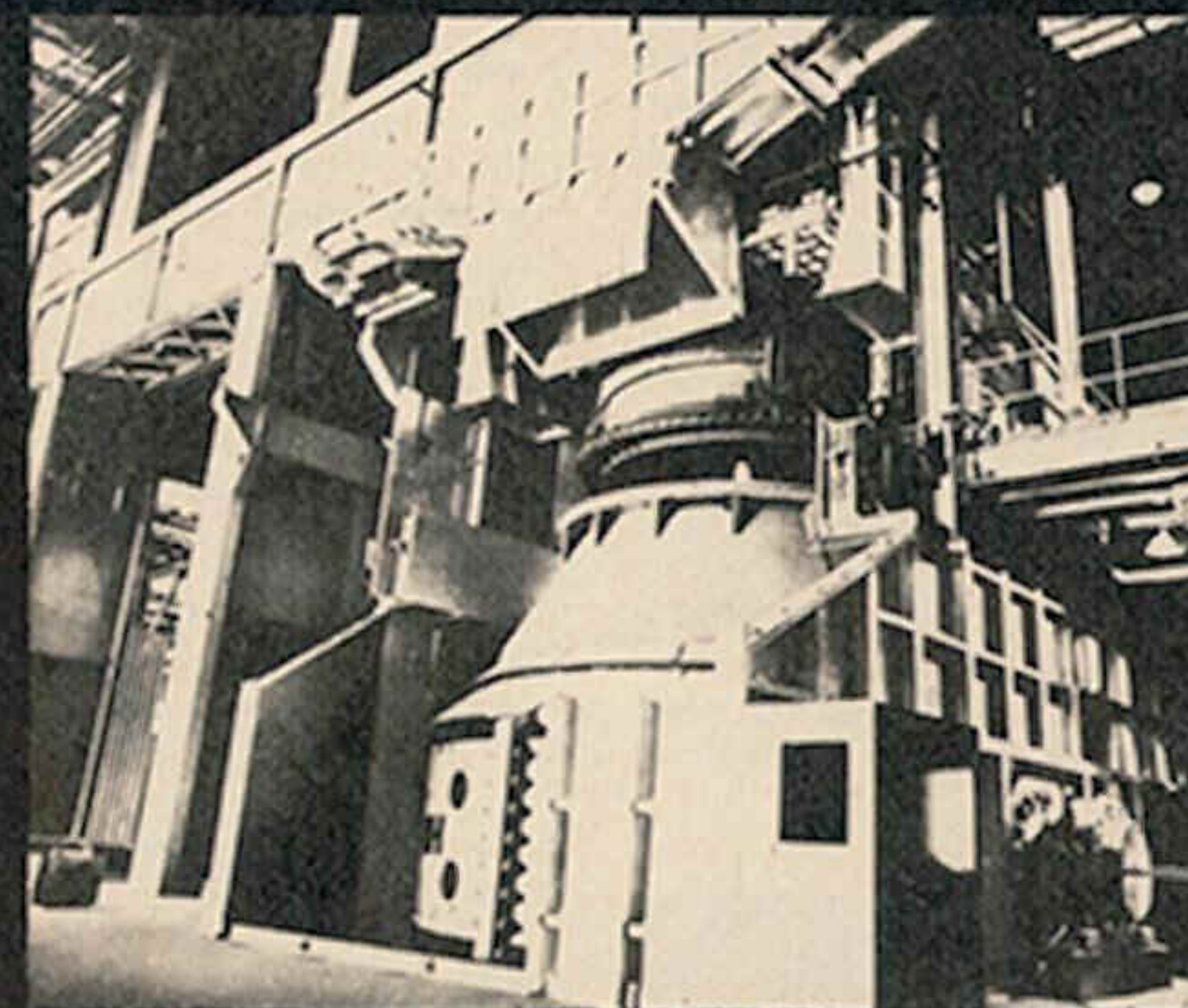
Uno de los convertidores de 160/183 t. de capacidad.
