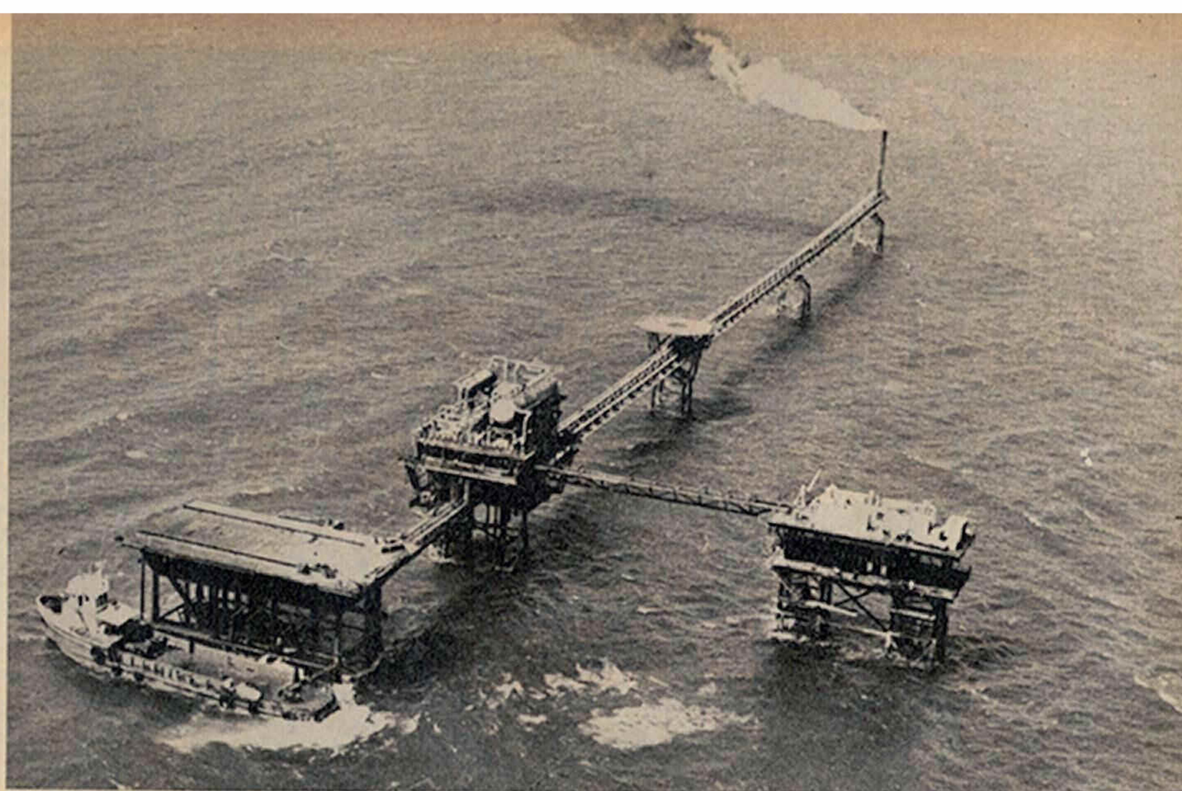
TORRE DE EXPLOTACION EN ALTA MAR Sólo un par de empresas tiene la tecnología
