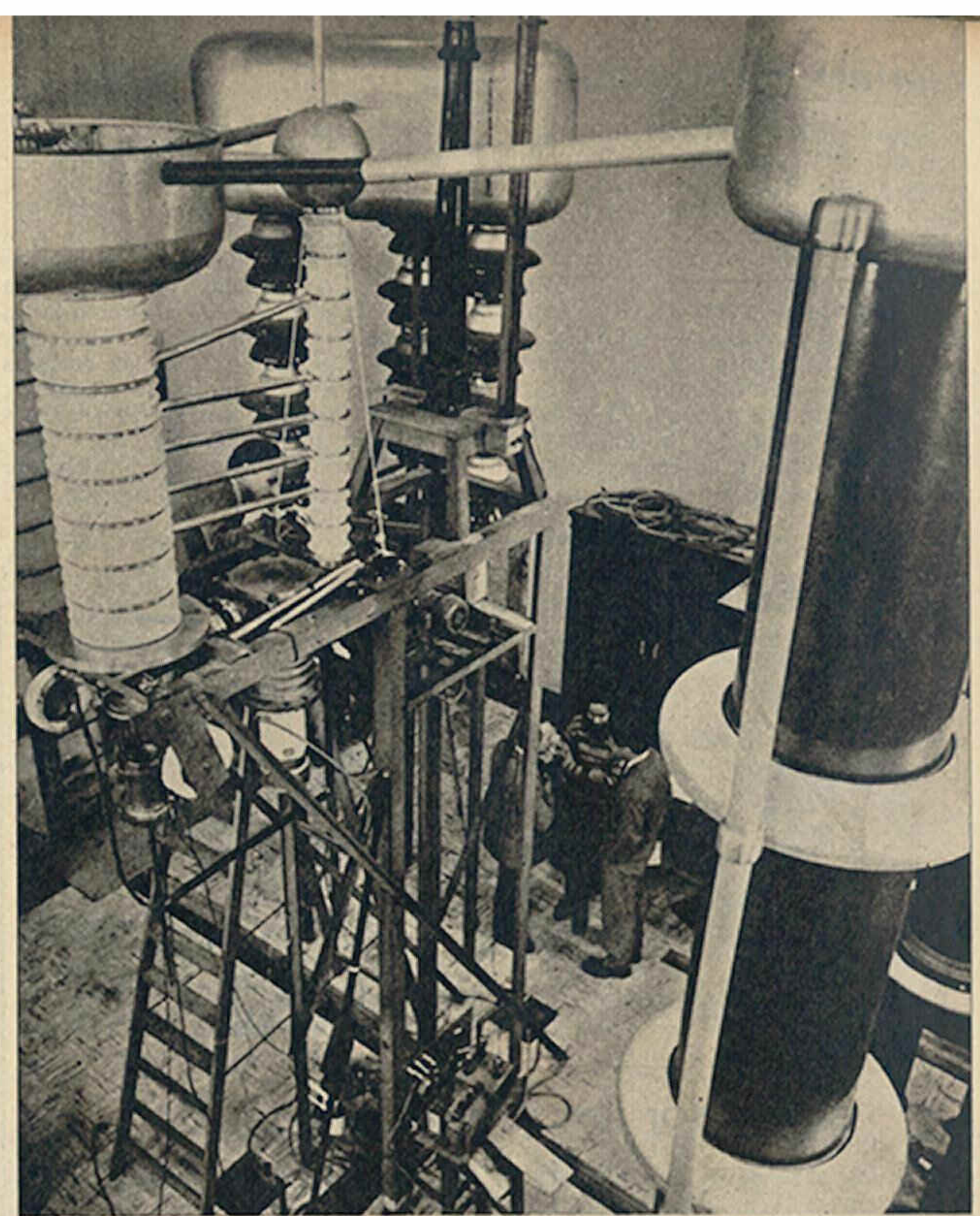
Acelerador de iones en el Centro Atómico Bariloche: Investigación básica avanzada.
