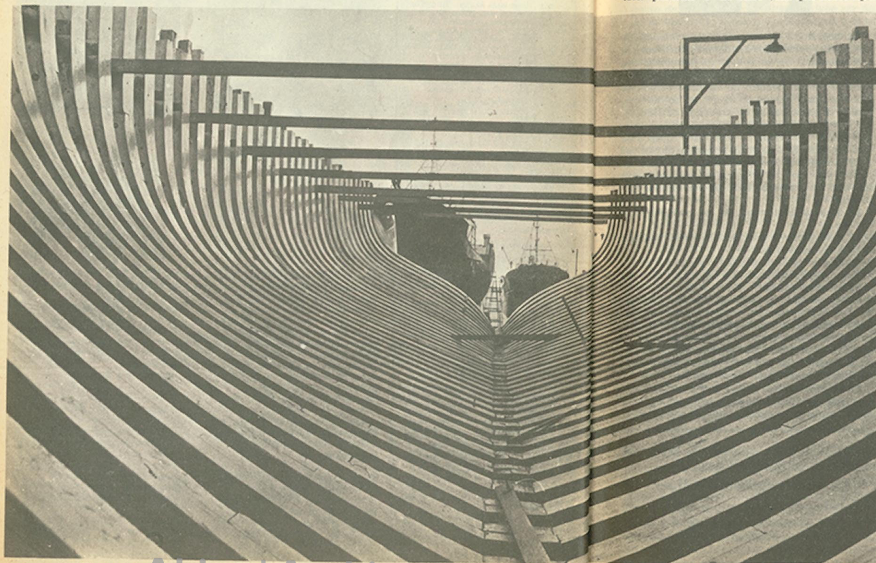
Un casco en los astilleros argentinos. El aporte de elevada tecnología permite un óptimo nivel de calidad y diversificación productiva.
