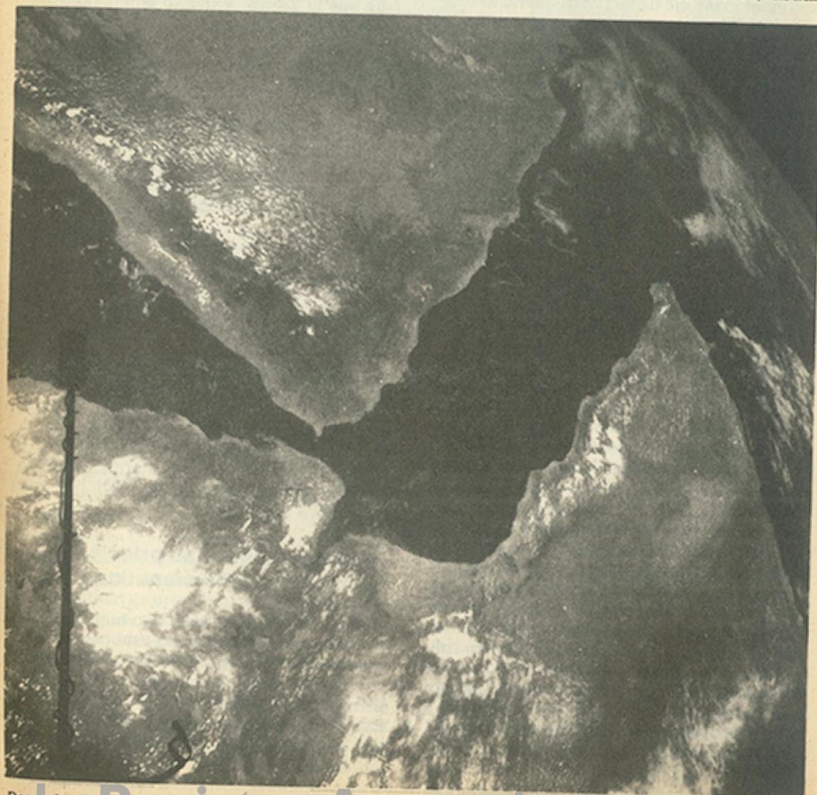
Desembocadura del Mar Rojo desde un satélite. 1960 marca el retorno del mundo a la era neoboreal.
