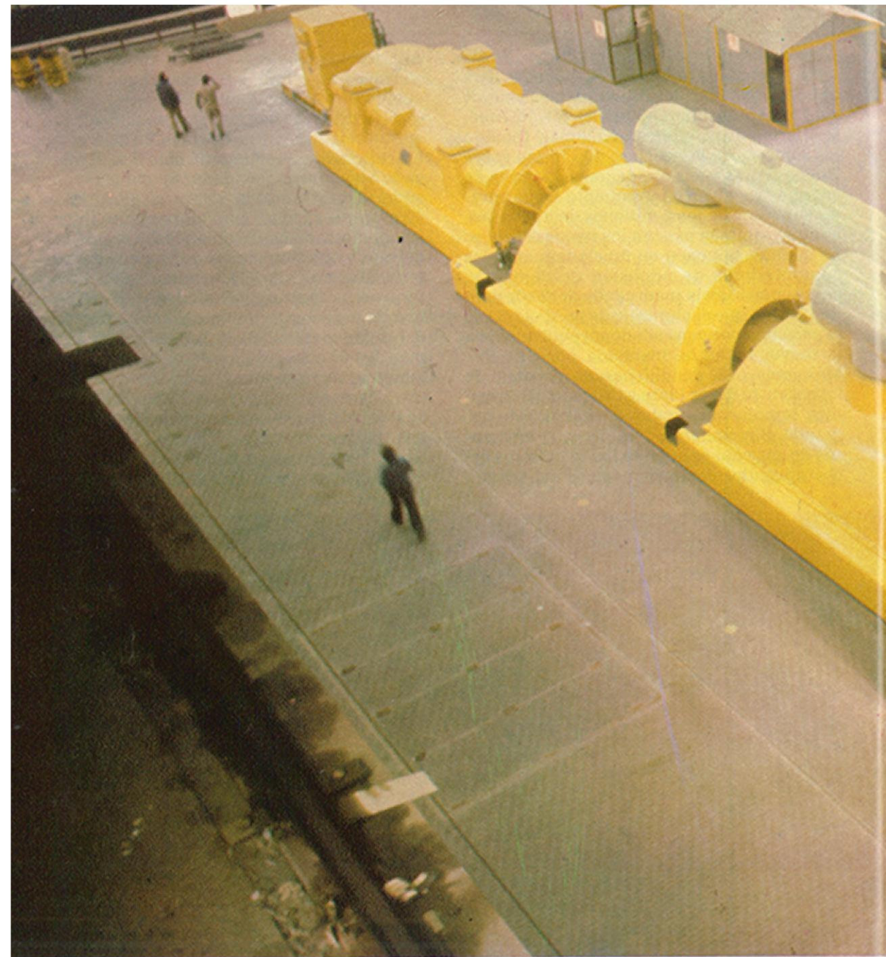
Turboalternador N° 6, generador de una potencia de 350 mil kilovatios, el de mayor magnitud
