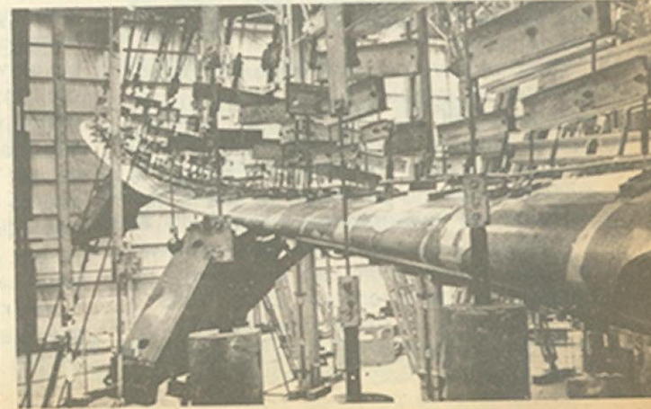
Buscando la "caja negra". El ala de un jet sometida a un terrible ensayo.
